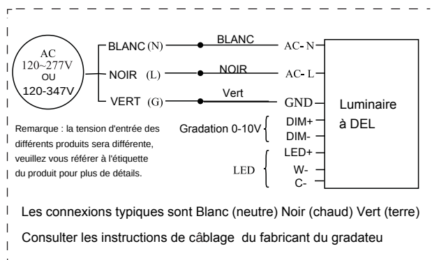
schémas de câblage
